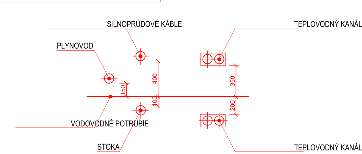
Tabulka 1. NAJMENŠIE DOVOLENÉ VODOROVNÉ VZDIALENOSTI PRI SÚBEHU PODZEMNÝCH VEDENÍ 1) (rozmery sú v cm) – STN 73 6005.
