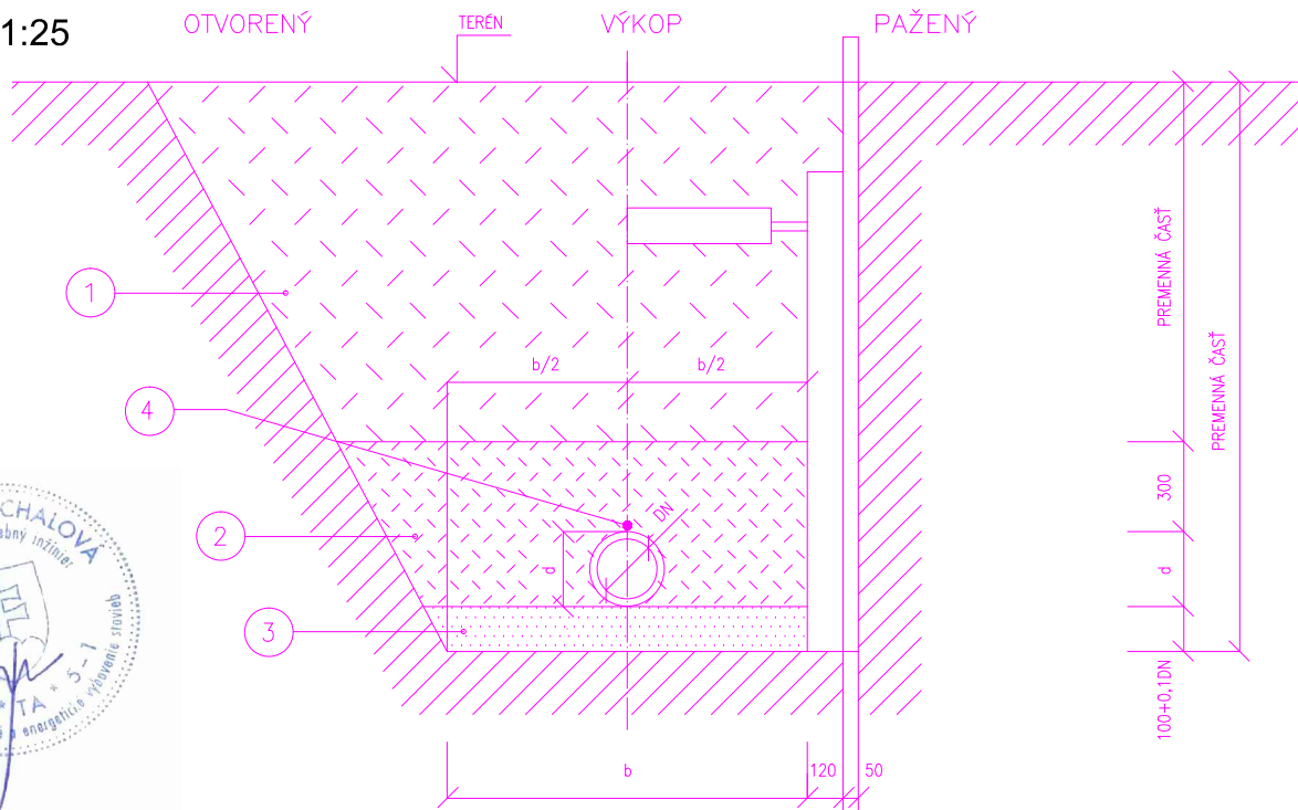
ŠÍRKA DŇA VÝKOPU PRI KLADENÍ POTRUBIA
