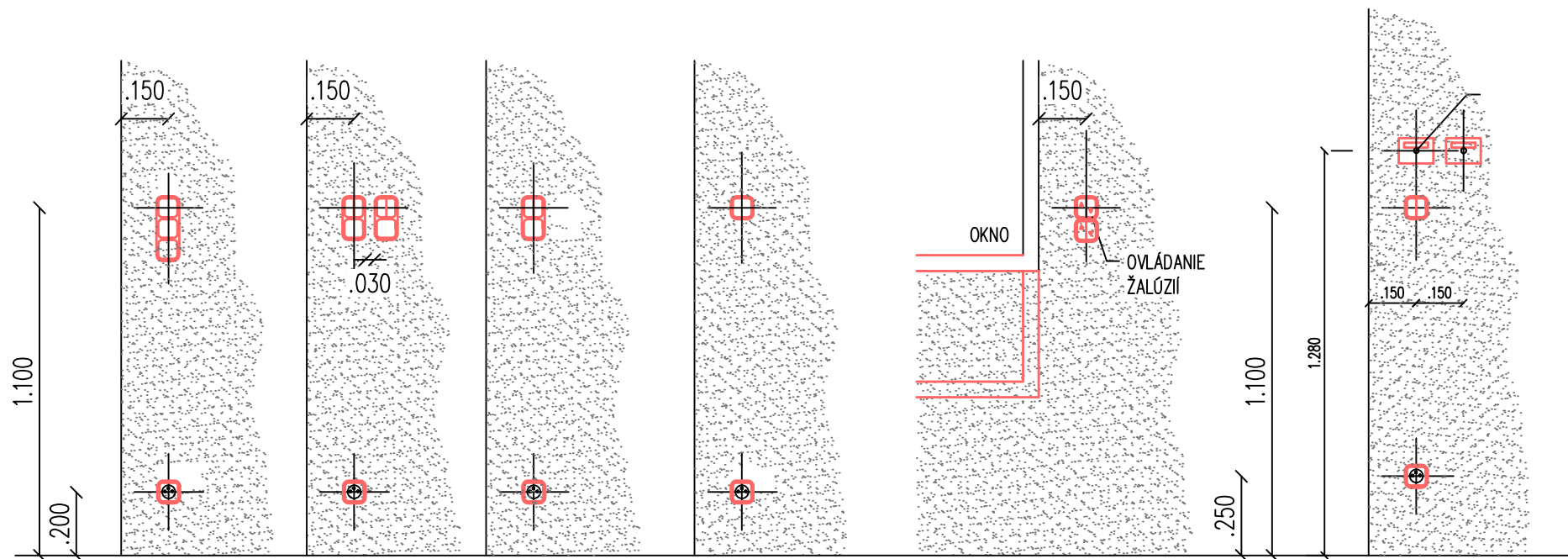
Inštalovanie ovládania (klimatizácie) termostátov podlahových konvektorov vypínačov
