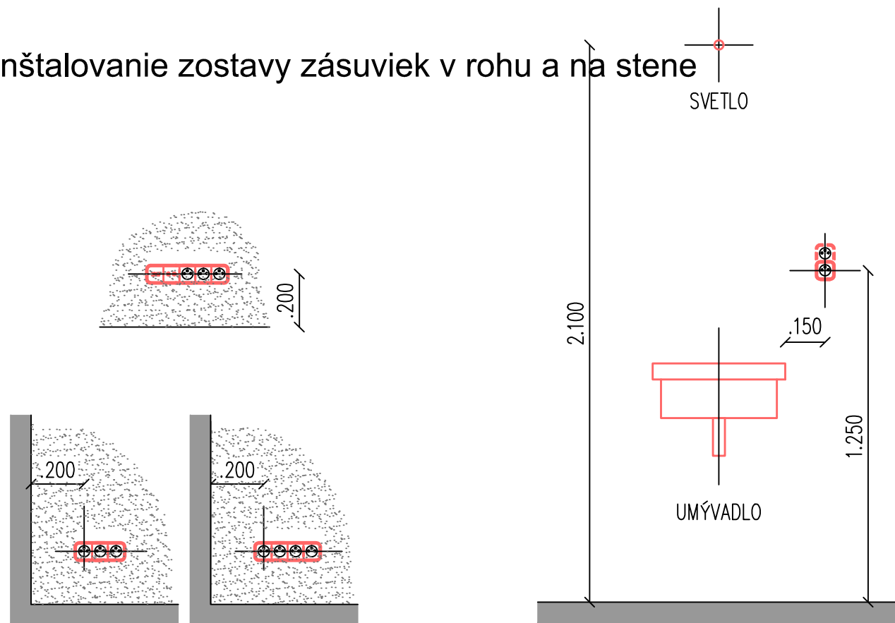
Inštalovanie zásuviek pri umývadle
