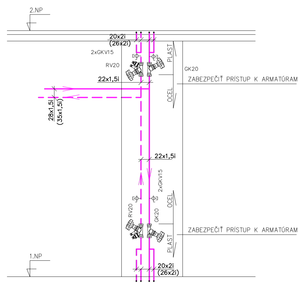
DETAIL VEDENIA POTRUBIA V ŠACHTE
