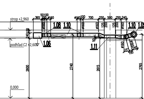
REZ B–B
