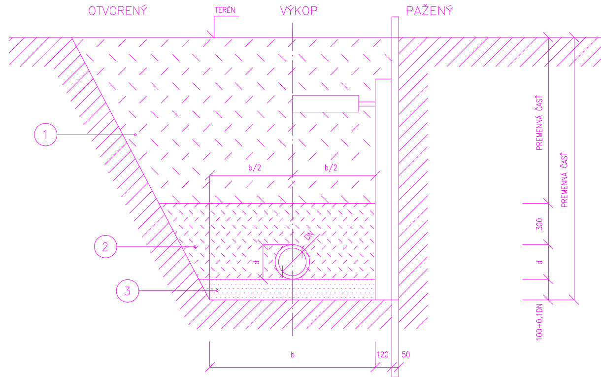
ŠÍRKA DNA VÝKOPU PRI KLADENÍ POTRUBIA
